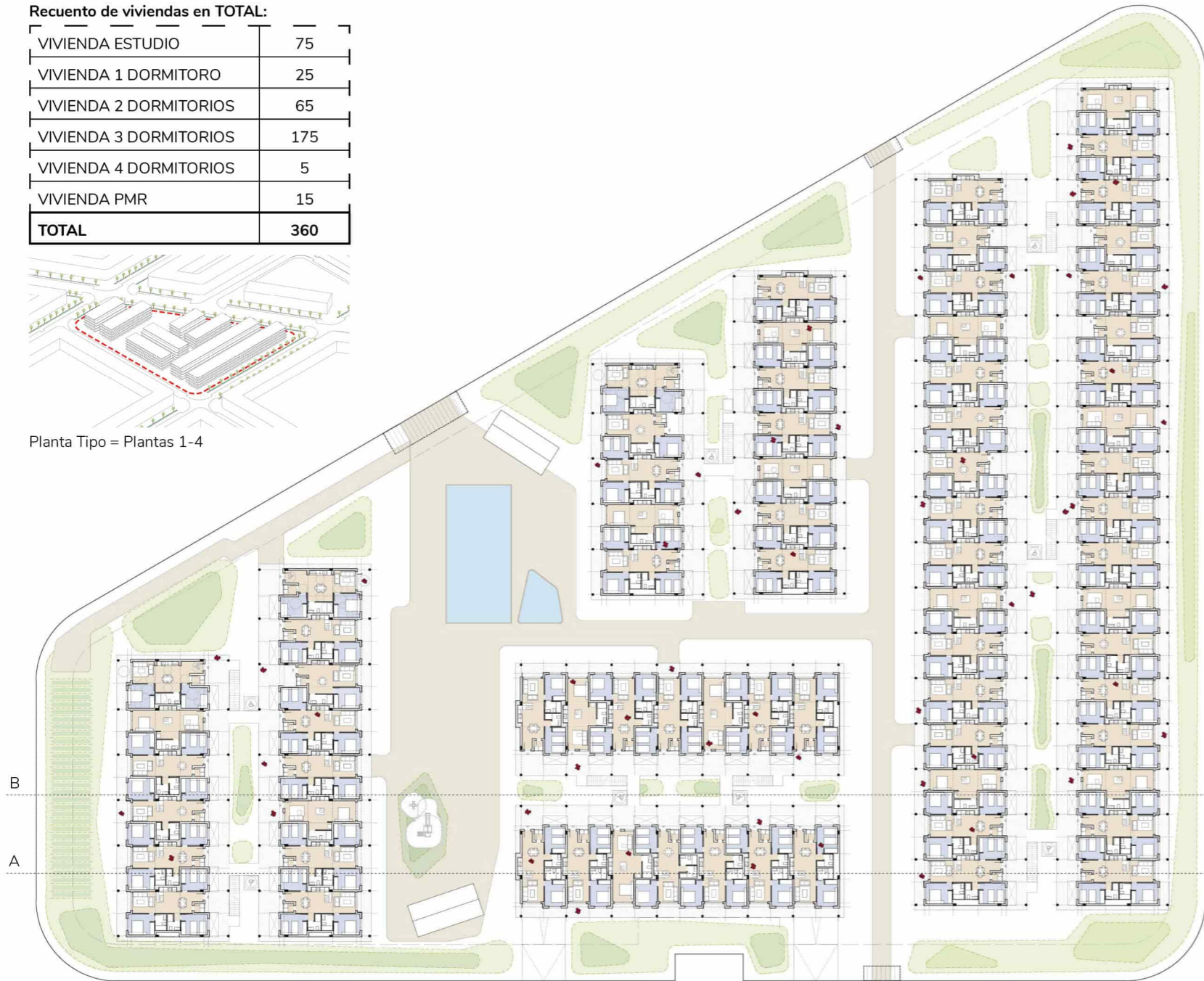
Planta Tipo E: 1/750
