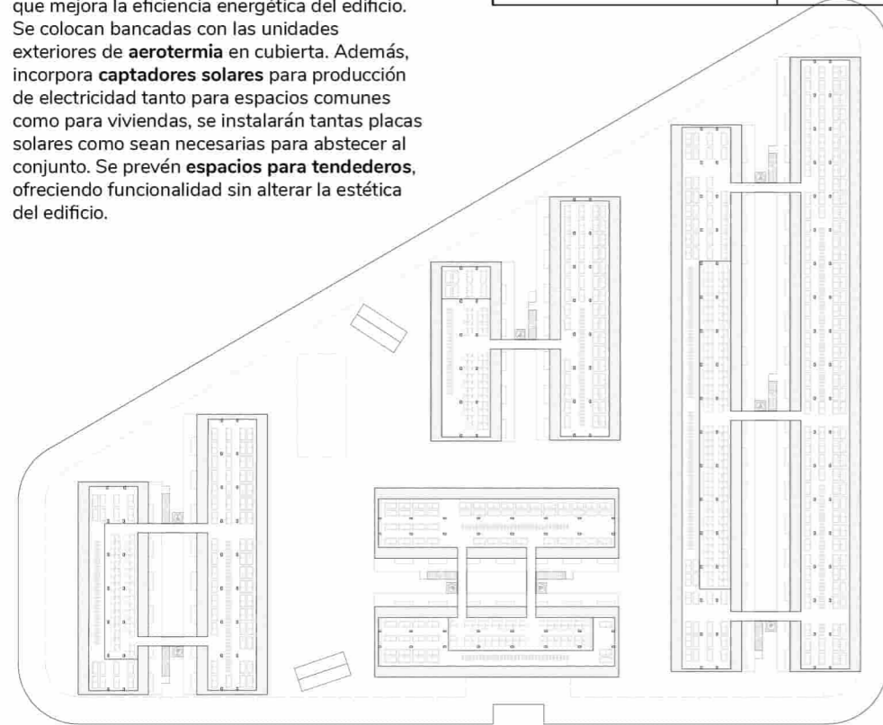
Planta de Cubiertas E: 1/1.250
